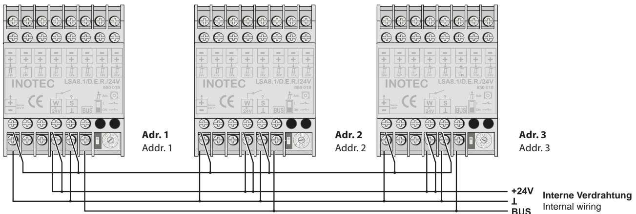
Potentialfreie Eingänge 24V Potential-free inputs 24V
