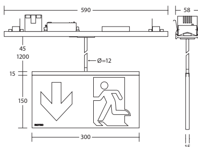
BNP 9100 P Ino-Traq BNP 9100 P Ino-Traq
